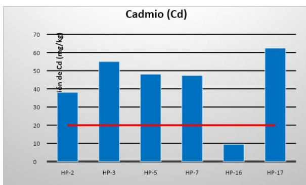
Figura 9. Concentración de cadmio en las muestras de jales de la mina La Prieta-Chihuahua.
