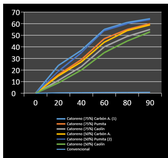
Figura 7. Porcentaje de biodegradación
