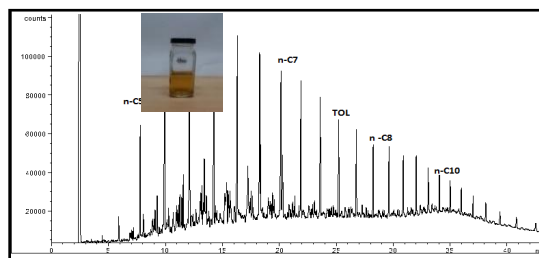
Figura 1. Análisis por CG del agua residual sin modificar el camalote
