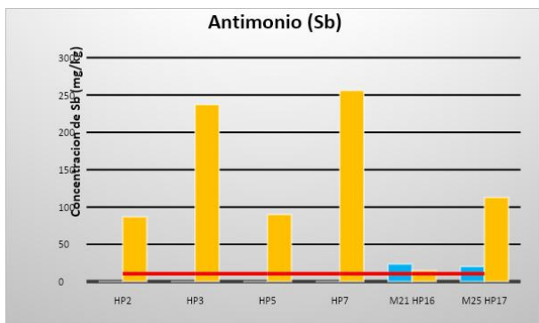
Figura 6. Concentraciones de antimonio en las muestras de jales de las minas Cerro de Mercado-Durango y La Prieta-Chihuahua.
