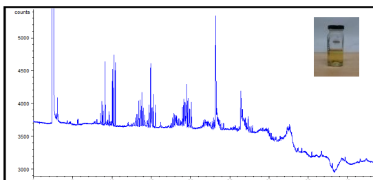
Figura 2. Análisis por CG del agua residual modificando el camalote con \text{Al}_2(\text{SO}_4)_3
