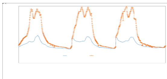
Fig. 6. Evolución de la temperatura del aire dentro y fuera del secador
