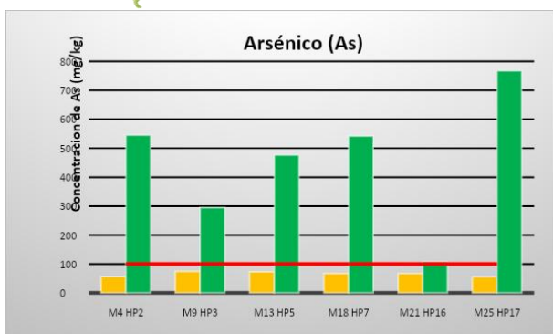
Figura 4. Concentraciones de arsénico en las muestras de jales de las minas Cerro de Mercado-Durango y La Prieta-Chihuahua.
