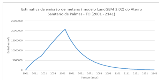
Figura 2: Estimativa da emissão de metano (modelo LandGEM 3.02) do Aterro Sanitário de Palmas – TO (2001 – 2141). Fonte: IBGE. Censo Demográfico 1991, 2000 e 2010; Projeção Populacional do PMSB de Palmas - TO; Modelagem matemática gerada pelo Software LandGEM.
