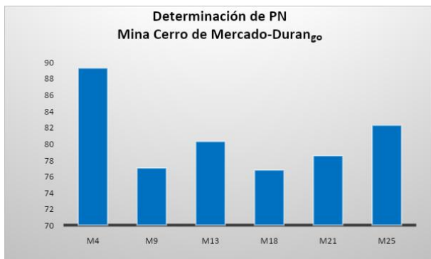
Figura 2. Determinación de potencial de neutralización de las muestras de jales de la mina Cerro de Mercado-Durango.
