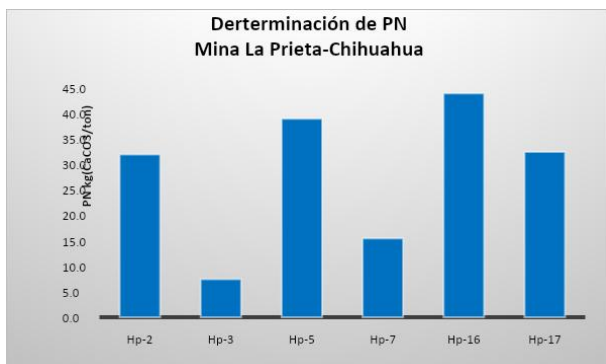
Figura 3. Determinación de potencial de neutralización de las muestras de jales de la mina La Prieta-Chihuahua.
