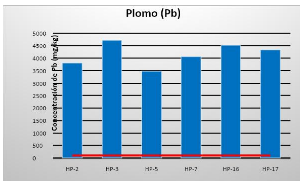
Figura 8. Concentración de plomo en las muestras de jales de la mina La Prieta-Chihuahua.
