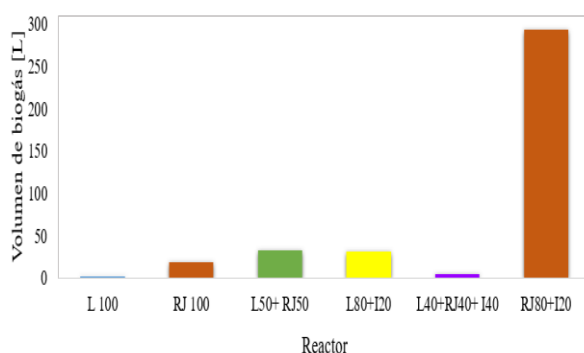
Figura 6. Volumen de biogás generado por reactor
