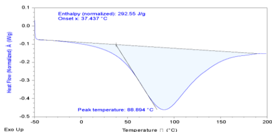
Figura 5. Gráfico del poder calorífico por DSC
