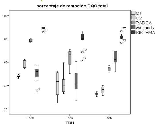
Figura 1. Porcentajes de remoción de DQO_{Total} en cada componente del sistema.
