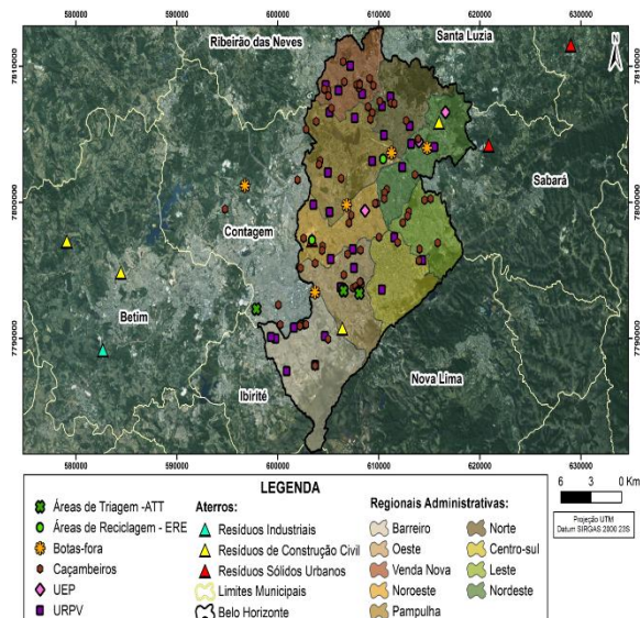
Figura 1. Distribuição e localização de equipamentos e instalações de gestão de RCC em BH e região (2016)
