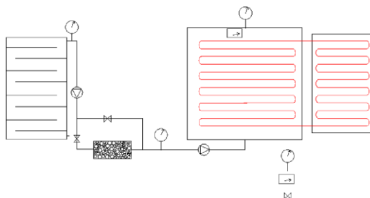
Fig.1. Diagrama esquemático del secador solar y el almacenador de calor
