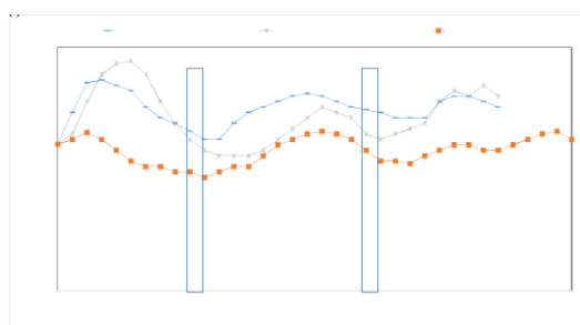
Fig. 4. Evolución de la temperatura del lodo del lodo sometido a procesos de secado
