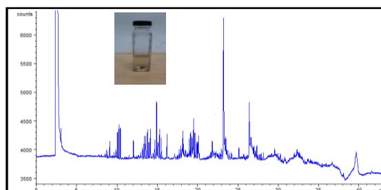
Figura 3. Análisis por CG del agua residual de mar.
