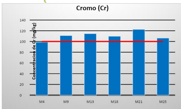
Figura 7. Concentración de cromo en las muestras de jales de la mina Cerro de Mercado-Durango.
