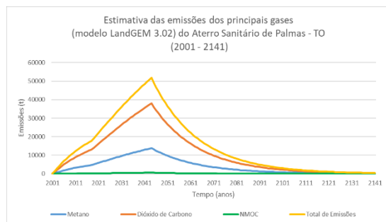
Figura 1: Gráfico da estimativa das emissões dos principais gases (modelo LandGEM 3.02) do Aterro Sanitário de Palmas – TO (2001 – 2141). Fonte: IBGE. Censo Demográfico 1991, 2000 e 2010; Projeção Populacional do PMSB de Palmas - TO; Modelagem matemática gerada pelo Software LandGEM.
