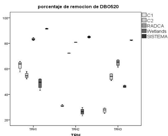
Figura 2. Porcentajes de remoción de DBO_{5-20} en cada componente del sistema.
