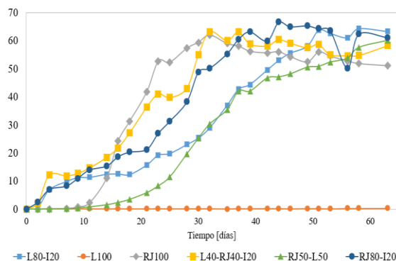
Figura 5. Producción de metano en los reactores
